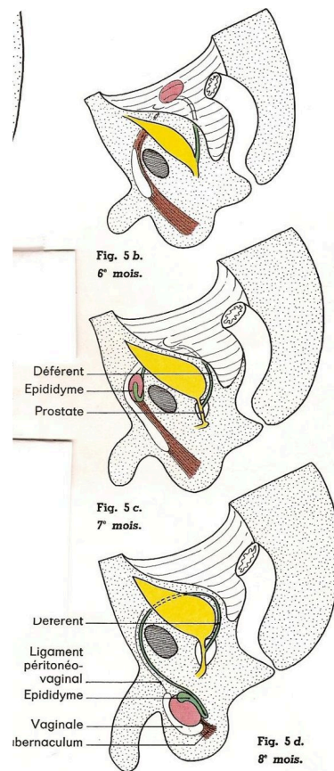
Fig. 5. — Migration testiculaire
